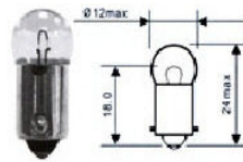
14401-A62 6V-3W 14402-A72 12V-3W
