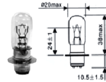
14452-A3625 6V-25/25W 14457-A3603 12V-25/25W 14469-A5228 12V-35/25W
