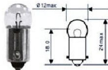
14401-A62 6V-3W 14402-A72 12V-3W
