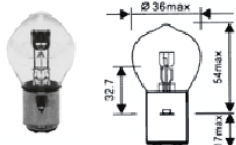
14416 (A7385) 12V-60/60W
